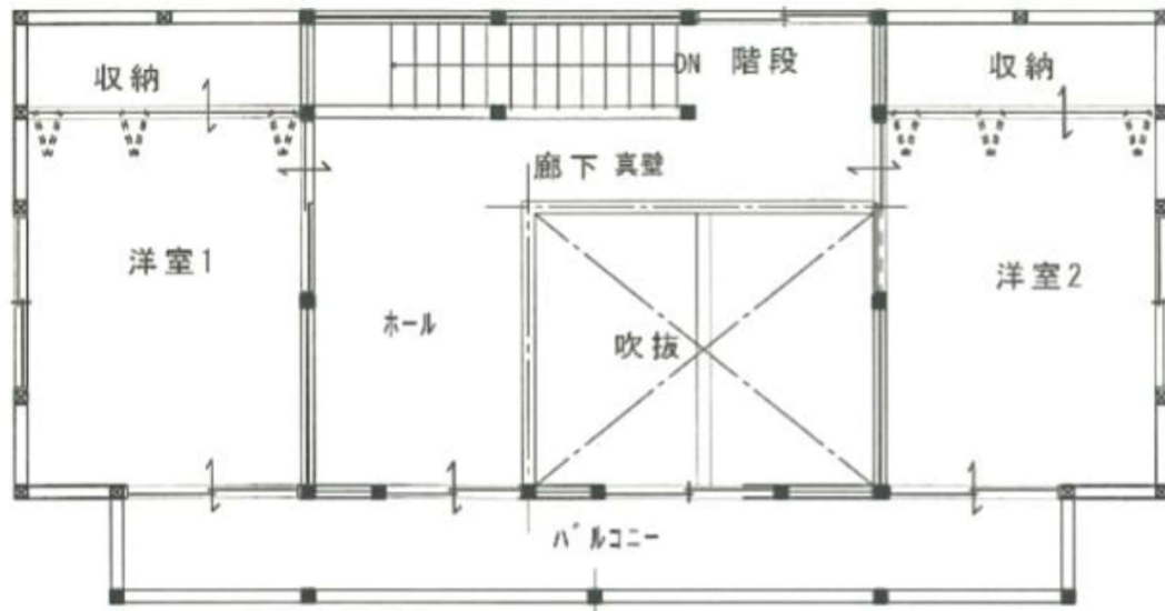
2階平面図
