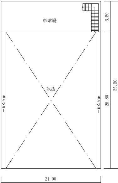
②1 屋内運動場 2 階平面図
