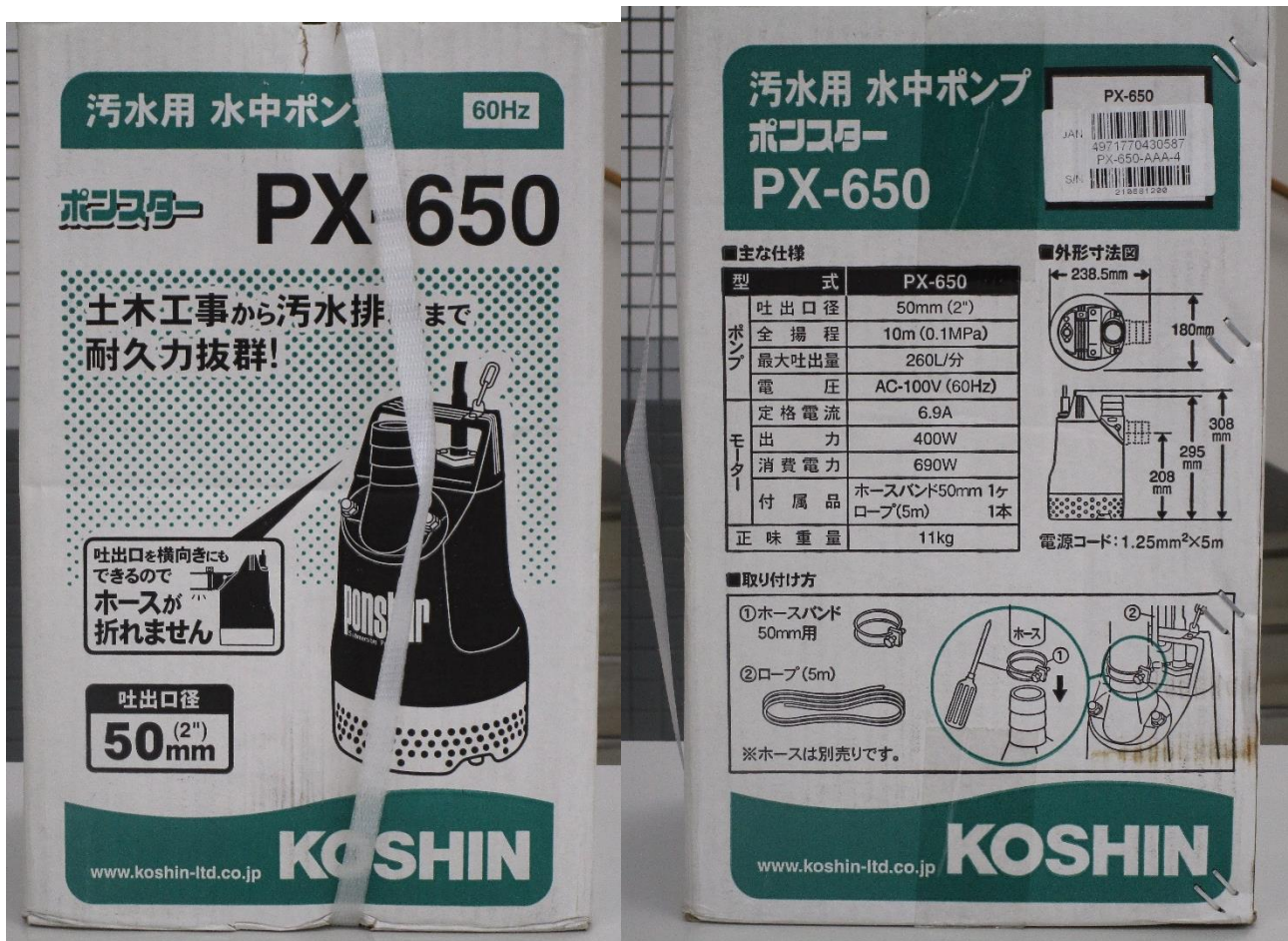
① KOSHIN 汚水用 水中ポンプ ポンスター PX-650
